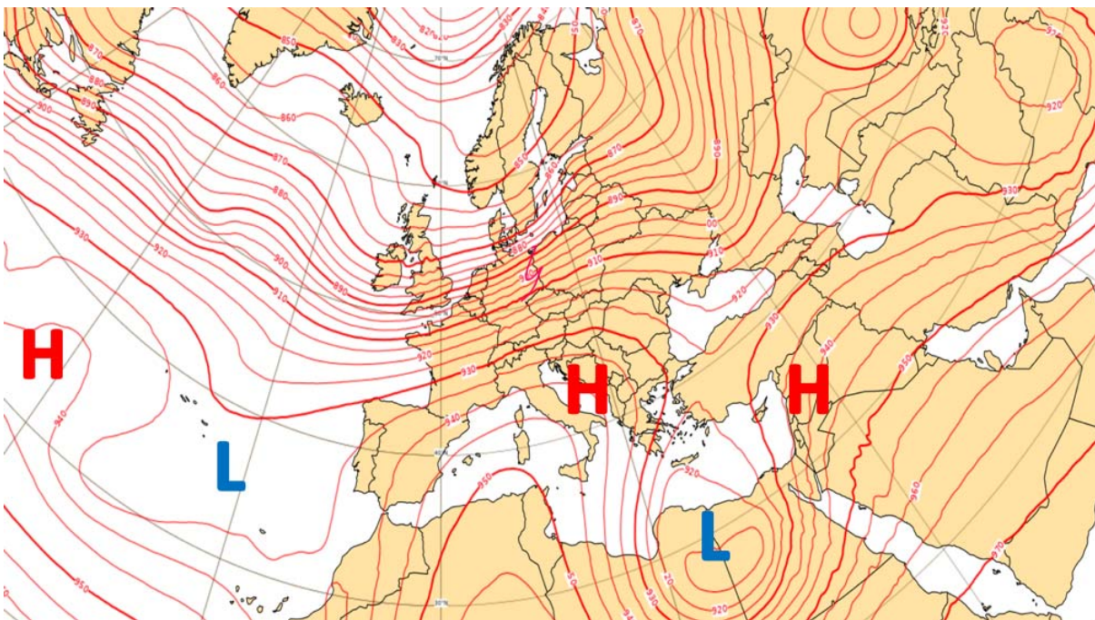
Χάρτης κατανομής συστημάτων ανώτερης ατμόσφαιρας στις 12/3/2020 στις 12:00 (Τοπική Ώρα)
